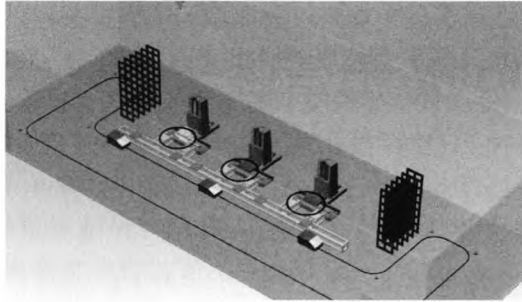
图 1 柔性生产线布局示意图
