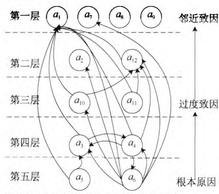
图5 柔性生产线系统故障致因因素递阶层次图模型
